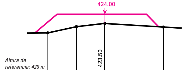
Perfil transversal 175
